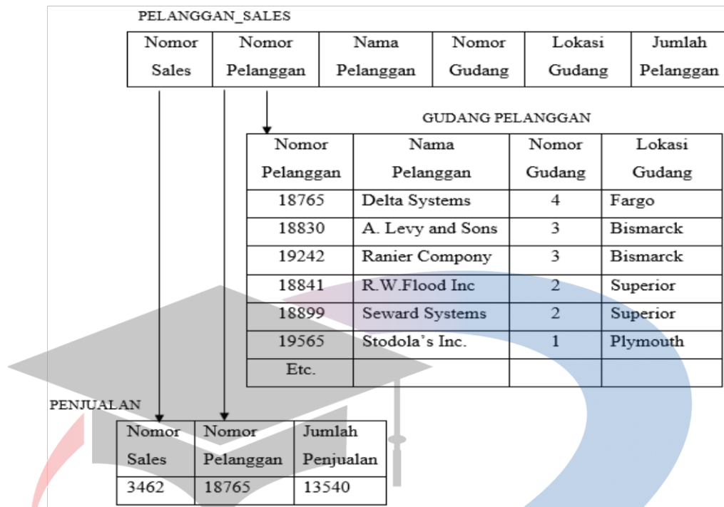
Gambar 2. 9 Contoh Bentuk Normalisasi Kedua
