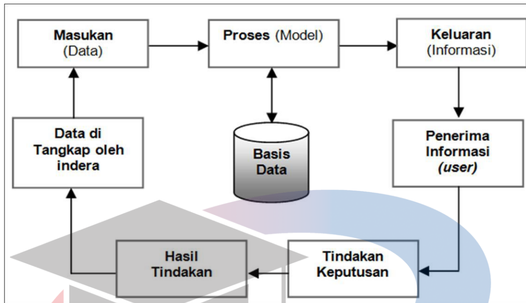
Gambar 2. 2 Siklus Informasi
