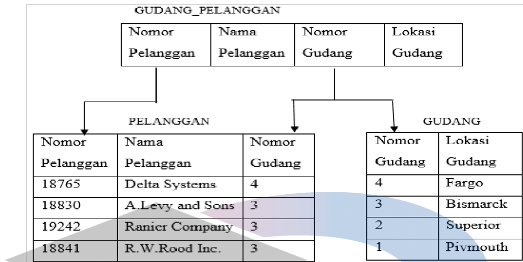
Gambar 2. 10 Contoh Bentuk Normalisasi Ketiga
