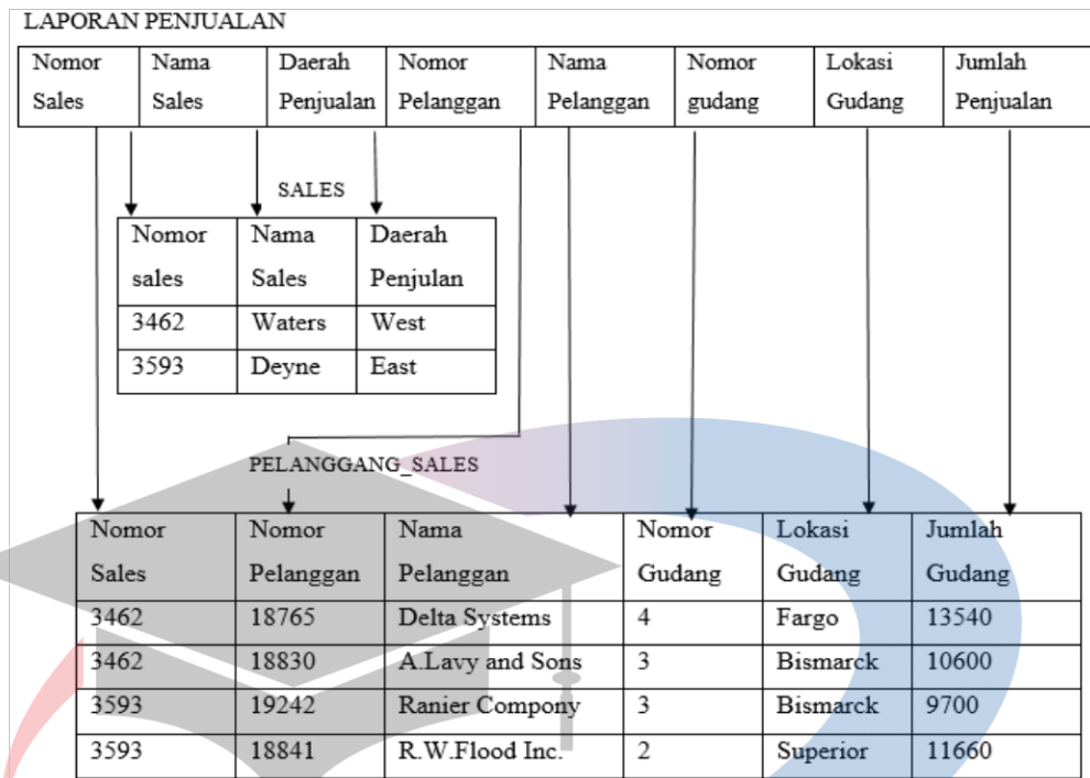
Gambar 2. 8 Contoh Bentuk Normalisasi Pertama
